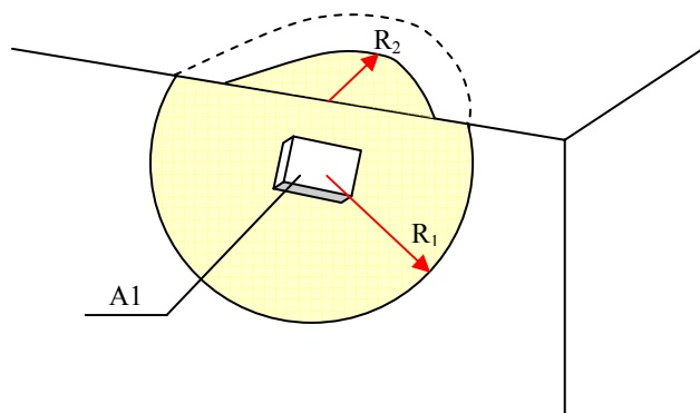
Рисунок 29 – Установка извещателей на монолитной конструкции с охватом 100 % охраняемой поверхности
