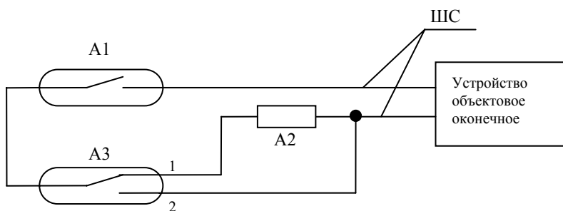
Рисунок 9 – Схема защиты магнитоcontactного извещателя от саботажа
